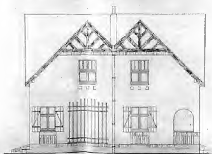
Vorder-Ansicht.
