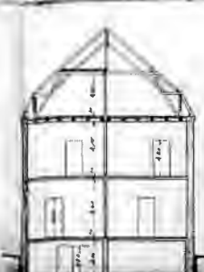
Schnitt 2-2
