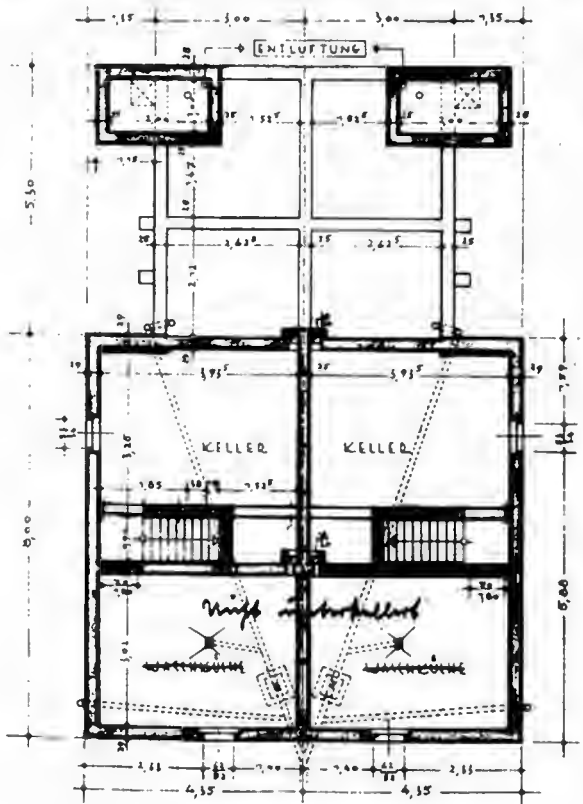
— KELLERGECHOSS —
