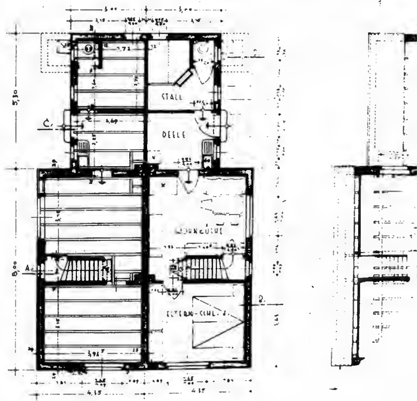
— ERDGECHOSS —
