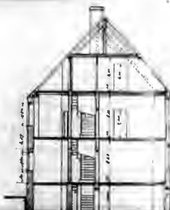
Schnitt 4-4
